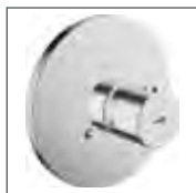
HANSA|LIVING Fertigmontageset mit Funktionseinheit Thermostat-Batterie, DN 20 (G3/4) passend zu HANSAVARIO- Einbaukörper* 0665 9105 verchromt ohne Mengenregulierung, Rosette rund, Ø 188 mm
