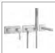
HANSAARONDA Fertigmontage- Installationspaket 1.5 Einhand-Batterie, DN 15 (G1/2) passend zu HANSAMATRIX Einbaukörper* 4487 2100 verchromt mit Brause-Set, mit Wanneneinlauf, DN 15
